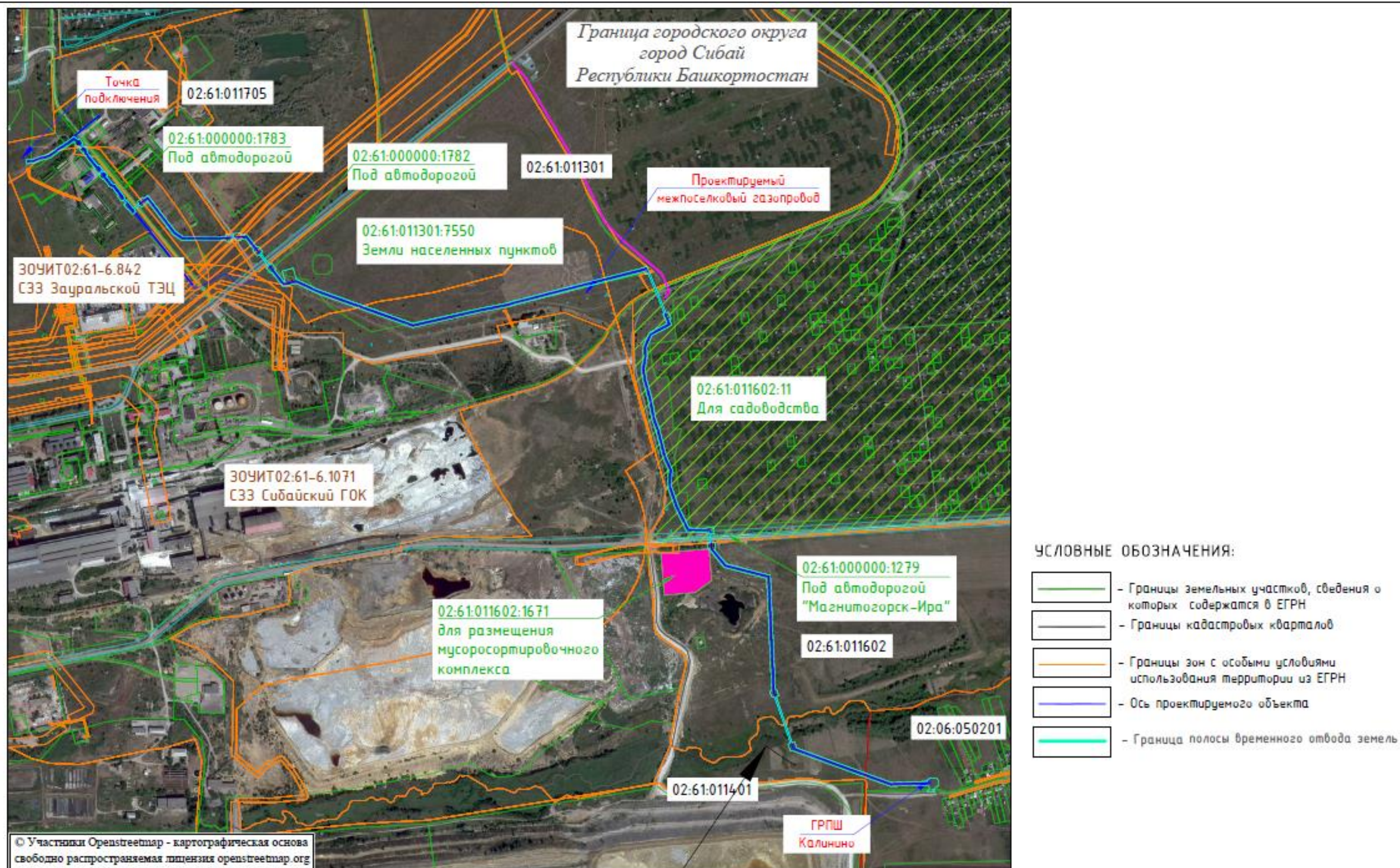
Рисунок 3.1 – Обзорная схема участка строительства
